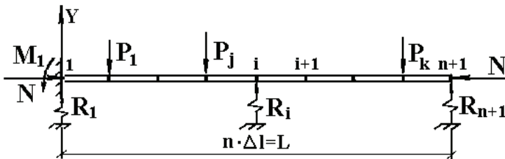
Рис. 1. Расчетная схема системы
