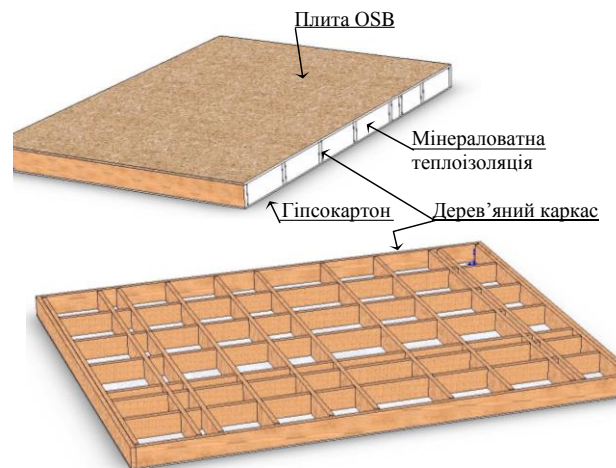
Рис. 1. Конструктивна схема дерев'яної плити / Construction scheme of wooden a plate
