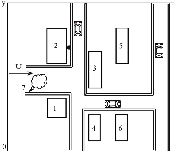
Рис.1. – Схема расчетной области: 1-6 – здания, 7 – место аварийного выброса
