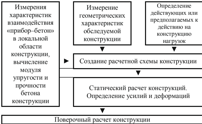
Рис. 1. Схема выполнения операций для осуществления проверочного расчета с использованием результатов определения прочности бетона методами неразрушающего контроля
