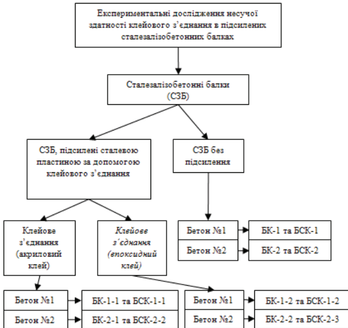
Рис.2. Схема експериментального дослідження з визначення несучої здатності клейового з'єднання та міцності і деформативності підсилені СЗБ
