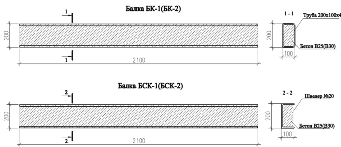
Рис.1 Зразки сталезалізобетонних експериментальних балок
