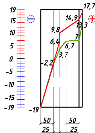
Рис. 5. Розподіл температур в перерізі огорожувальної конструкції з теплопровідним включенням (зеленим кольором вказана температура в місці розташування металевго профіля) /
