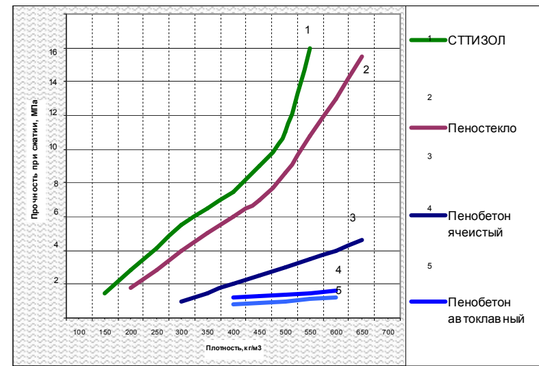
Рис. 1. Зависимость прочности при сжатии от плотности материалов
