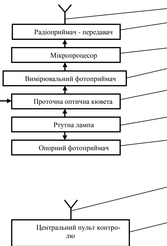
Рис. 1. Схема газоаналізатора
