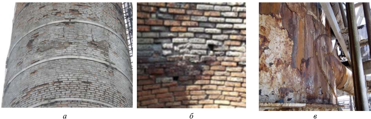
Рис. 2. Пошкодження димових труб: а – тріщини та руйнування окремих цеглин; б – вигін внутрішніх поверхонь; в – корозія конструкції /
