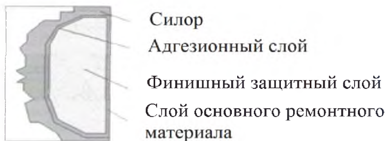
Рис. 1. Восстановление геометрии и упрочнение стеновых конструкций при помощи полимерной композиции "Силор"
