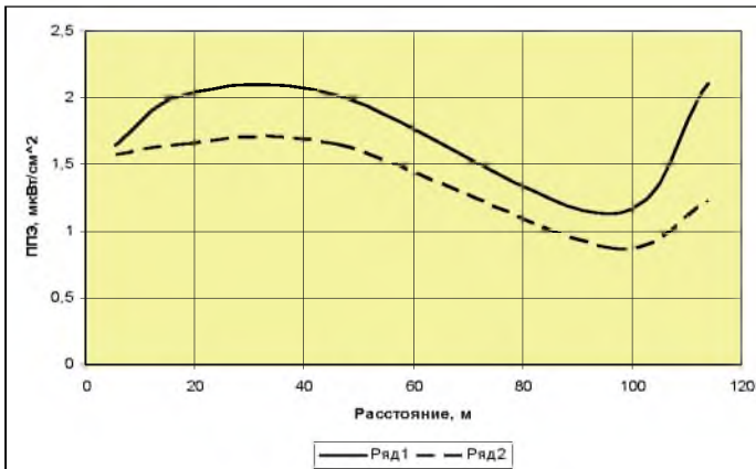
Рис.4. Зависимость плотности ЭМП от расстояния для частот сотовой связи: Ряд1 – 900МГц, Ряд2 – 1800МГц.
